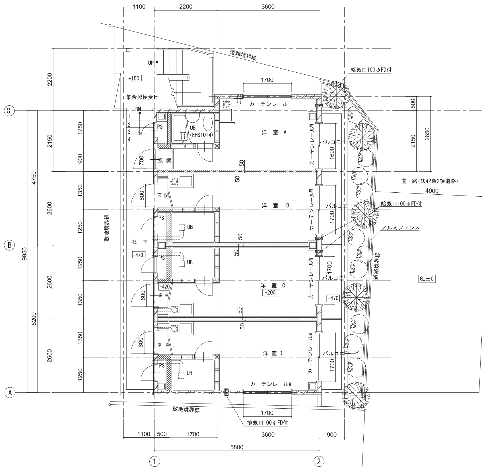
1F平面詳細図
